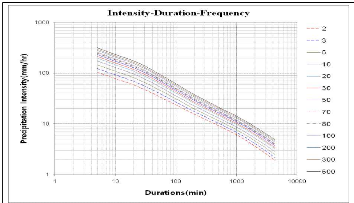
【그림 40.9】 균위지역 IDF곡선
