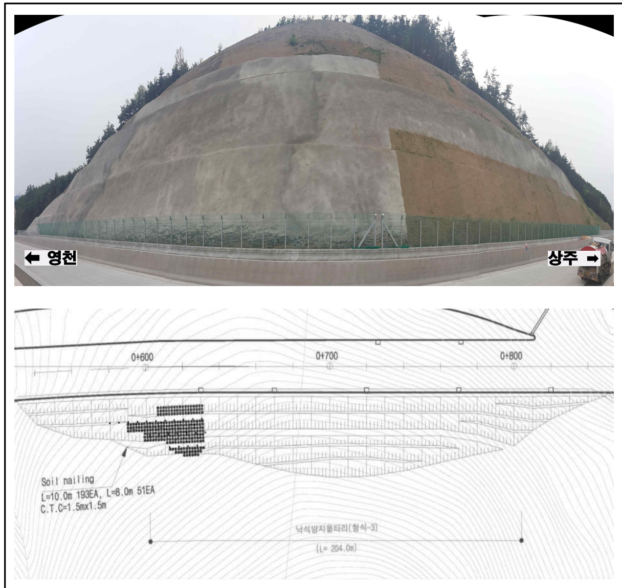
【그림 40.14】 영천절토40 검토대상 비탈면구간
